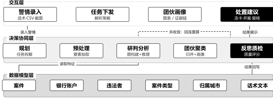
图1 系统三层架构（黑底为决策输出节点）
