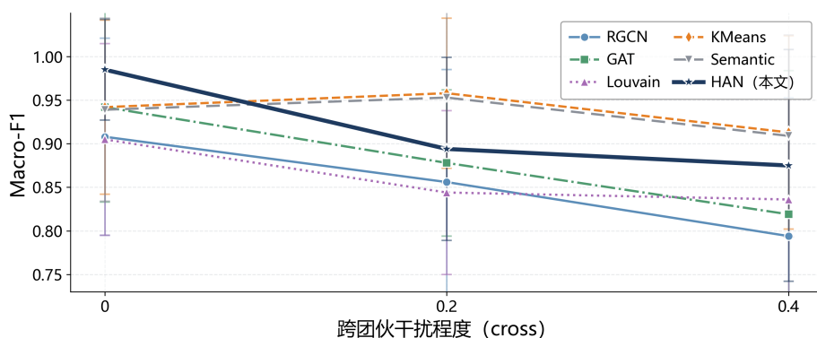
图3 同协议异构图基线在跨团伙干扰 \text{cross} \in \{0.0, 0.2, 0.4\} 下的 Macro-F1 曲线 (15 seeds, 误差棒为 std)。HAN 在 \text{cross}=0.0 最优；随干扰增大，特征基线 KMeans / Semantic 反超各图方法（诚实标注）。
