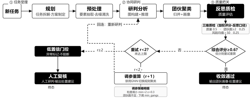
图 2 LangGraph 反思闭环编排（三维质检加权评分，未收敛回连重算，超限经低置信门控转人工复核）
