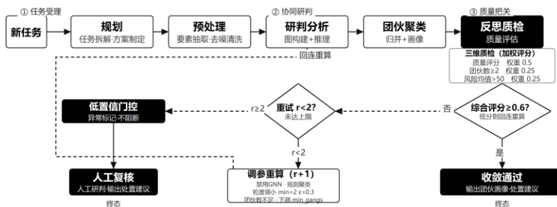
图 2 LangGraph 反思闭环编排（三维质检加权评分，未收敛回连重算，超限经低置信门控转人工复核）
