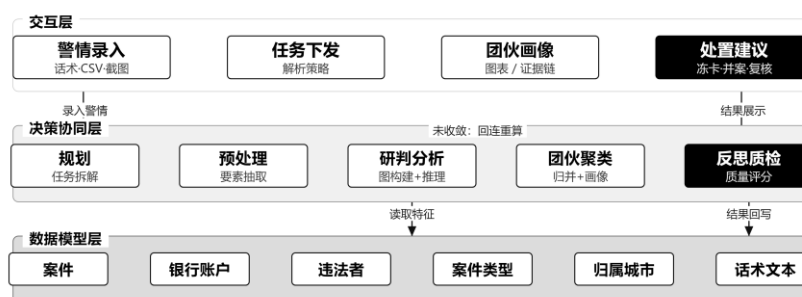
图 1 系统三层架构（黑底为决策输出节点）
