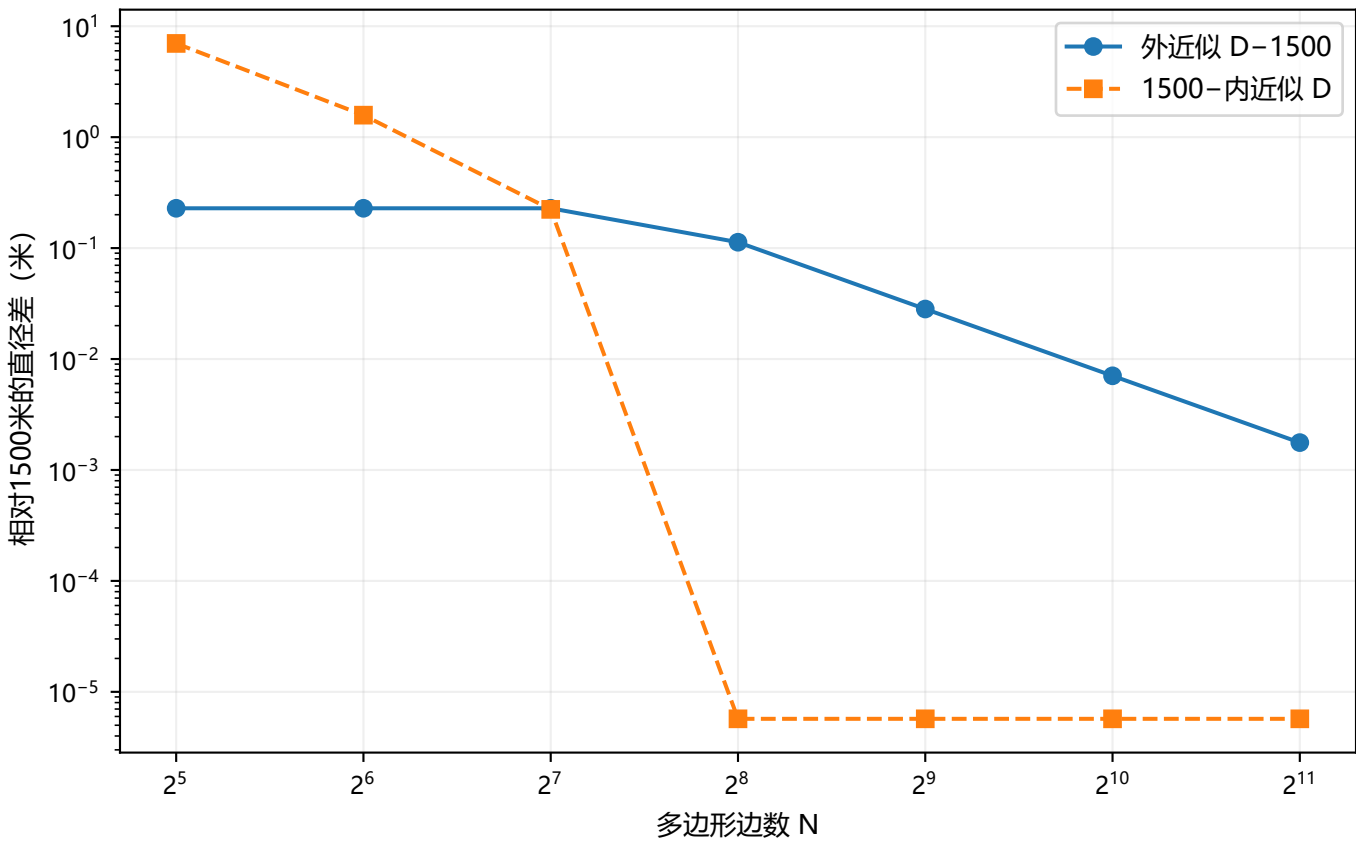
圆约束的内外逼近夹逼
