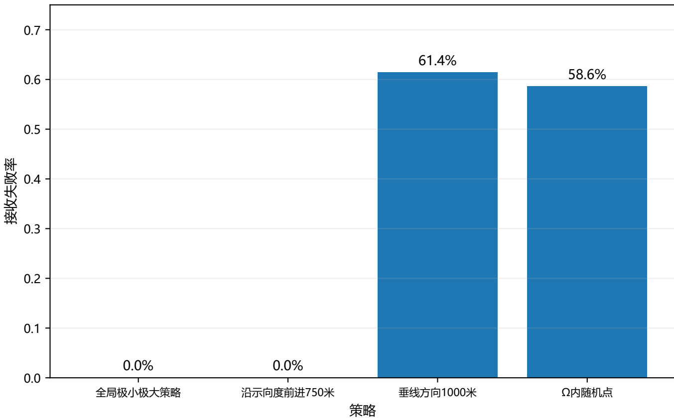
全部配对场景的接收失败率
