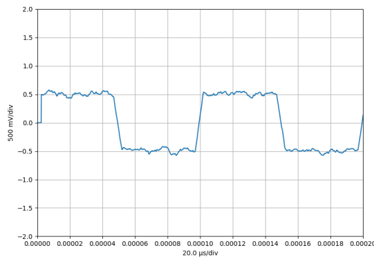
Abbildung 34: Signalverlauf rekursiver gleitender Mittelwertfilter (M=51) 10kHz Rechtecksignal mit überlagertem Rauschen (1Vpp; Bandbreite: 1MHz)
