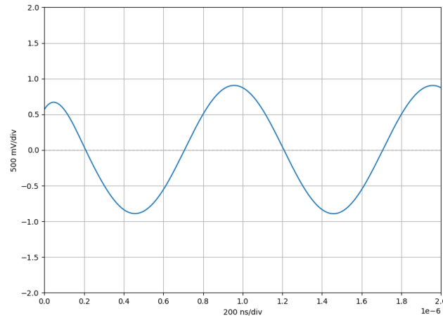
Abbildung 72: Testsignal: Sinus ( f = 1 MHz, V_{pp} = 2 V) Polynom-Interpolation
