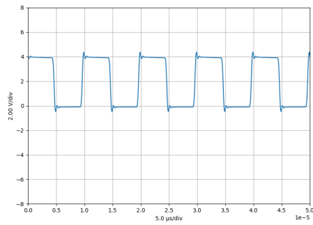
Abbildung 82: Testsignal: Rechteck ( f = 100 \text{ kHz} , V_{pp} = 4 \text{ V} ) V_{offset} = -0.77 \text{ V}
