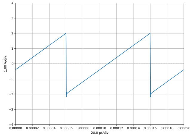
Abbildung 80: Testsignal: Sägezahn ( f = 10 \text{ kHz} , V_{pp} = 4 \text{ V} )
