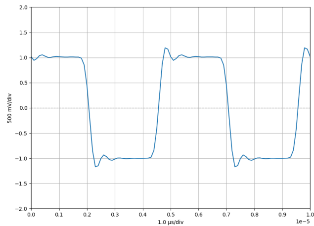
Abbildung 80: Testsignal: Rechteck ( f = 200 \text{ kHz} , V_{pp} = 2 \text{ V} )
