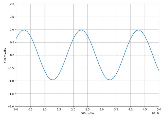
Abbildung 72: Testsignal: Sinus ( f = 500 \text{ kHz} , V_{pp} = 2 \text{ V} )
