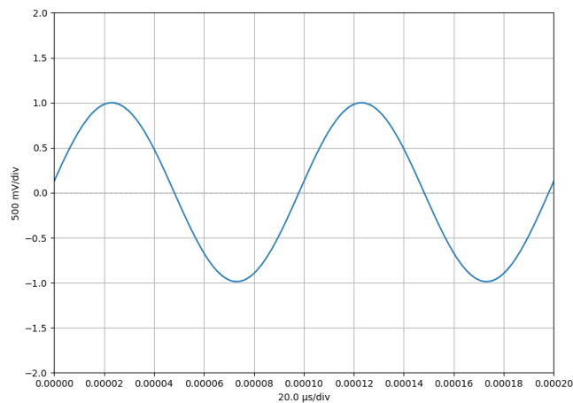
Abbildung 69: Testsignal: Sinus ( f = 10 \text{ kHz} , V_{pp} = 2 \text{ V} )
