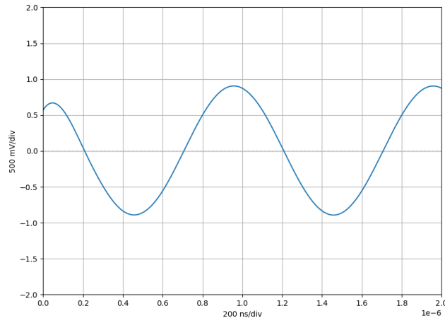
Abbildung 75: Testsignal: Sinus ( f = 1 MHz, V_{pp} = 2 V) Polynom-Interpolation
