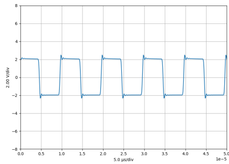
Abbildung 84: Testsignal: Rechteck ( f = 100 \text{ kHz} , V_{pp} = 4 \text{ V} ) V_{offset} = 0 \text{ V}
