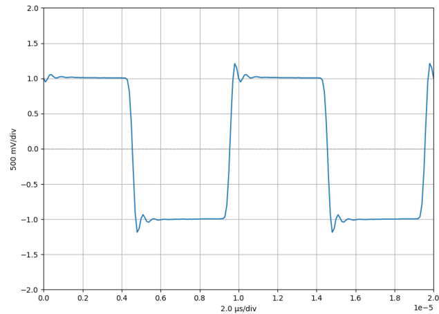
Abbildung 79: Testsignal: Rechteck ( f = 100 \text{ kHz} , V_{pp} = 2 \text{ V} )
