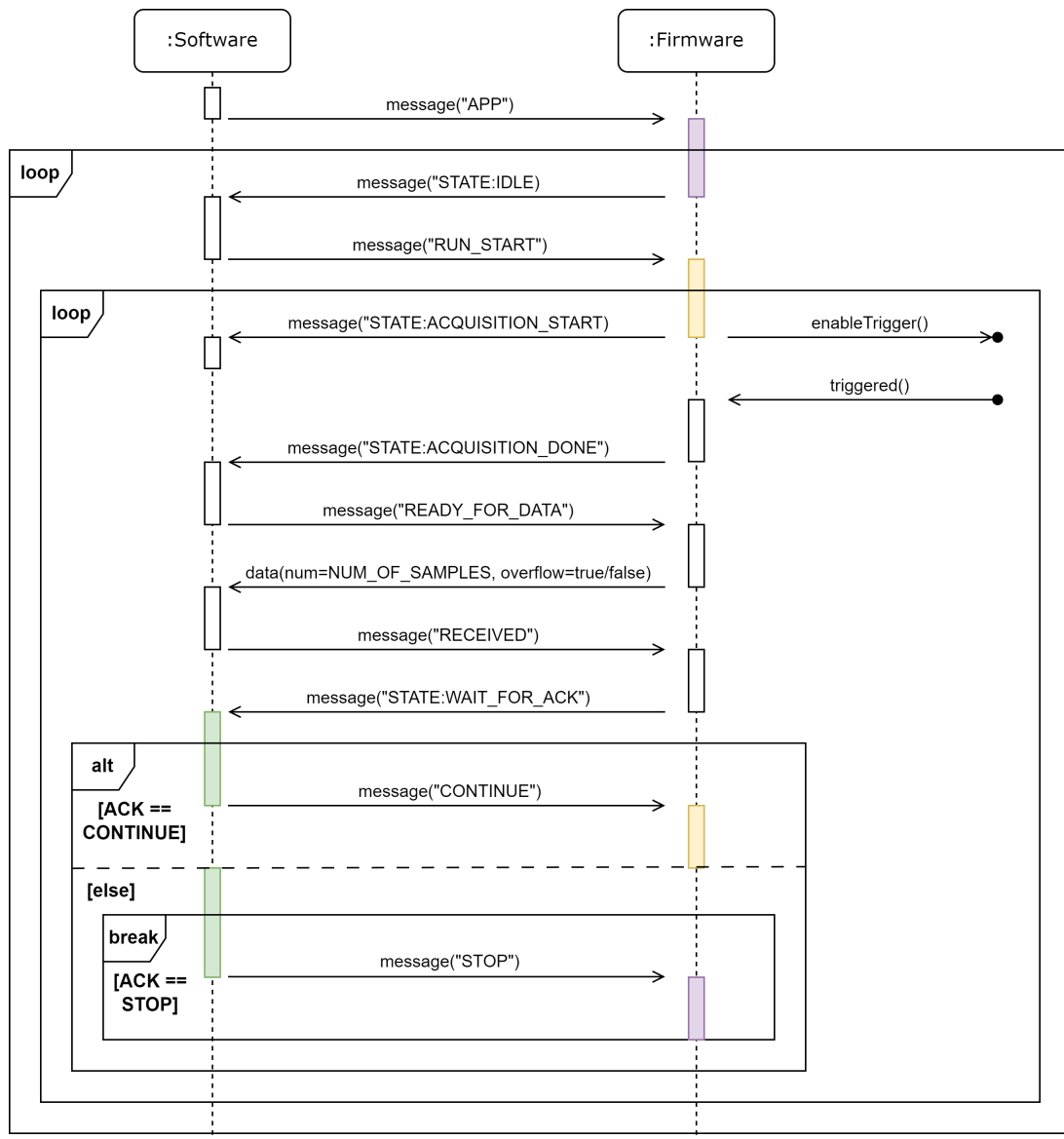
Abbildung 31: UML-Sequenzdiagramm: Kommunikation ohne Konfiguration
