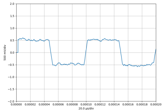
Abbildung 29: Signalverlauf kumulativer gleitender Mittelwertfilter (M=51) 10kHz Rechtecksignal mit überlagertem Rauschen (1Vpp; Bandbreite: 1MHz)
