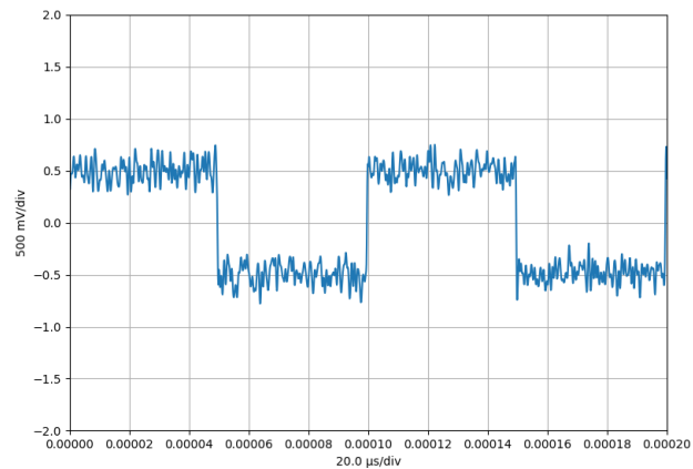
Abbildung 28: Signalverlauf ohne Filter 10kHz Rechtecksignal mit überlagertem Rauschen (1Vpp; Bandbreite: 1MHz)
