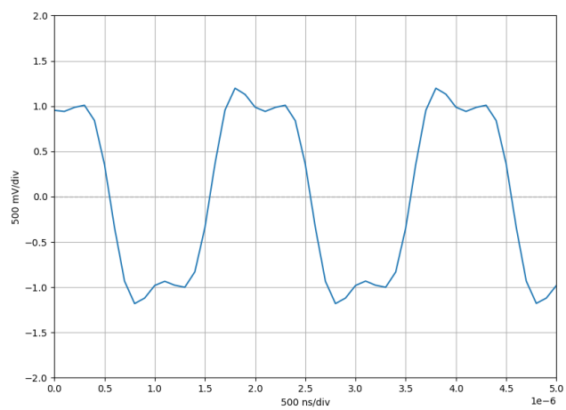
Abbildung 51: Testsignal: Rechteck ( f = 500 \text{ kHz} , V_{pp} = 2 \text{ V} )
