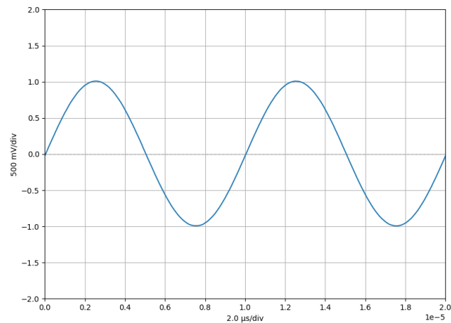
Abbildung 40: Testsignal: Sinus ( f = 100 \text{ kHz} , V_{pp} = 2 \text{ V} )
