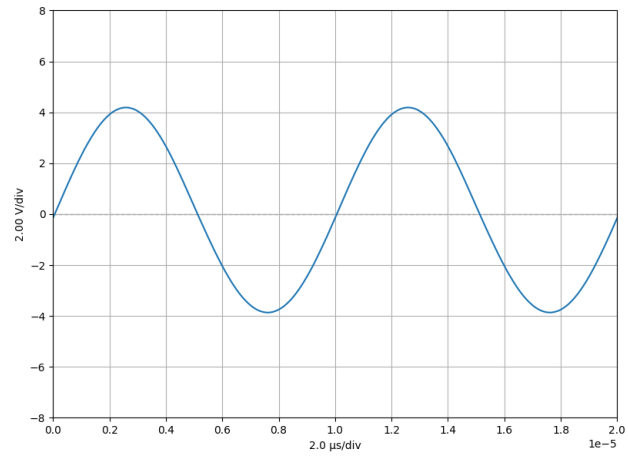
Abbildung 41: Testsignal: Sinus ( f = 100 \text{ kHz} , V_{pp} = 8 \text{ V} )
