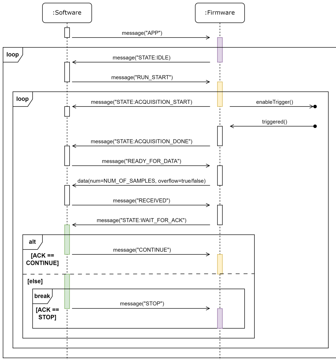
Abbildung 36: UML-Sequenzdiagramm: Kommunikation ohne Konfiguration
