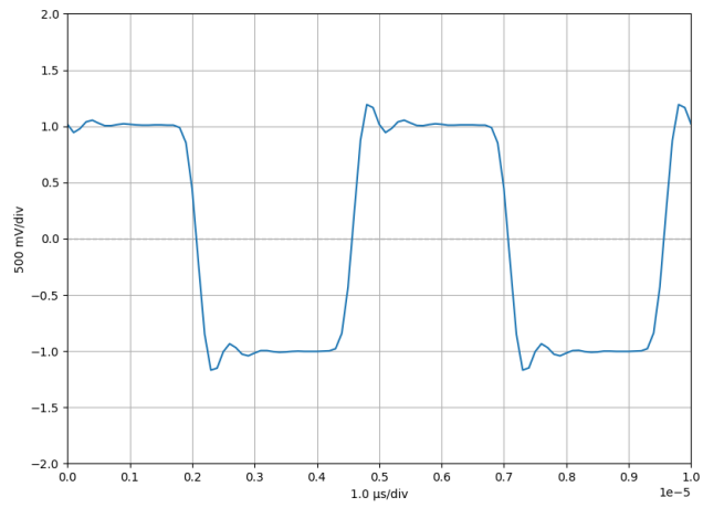
Abbildung 50: Testsignal: Rechteck ( f = 200 \text{ kHz} , V_{pp} = 2 \text{ V} )
