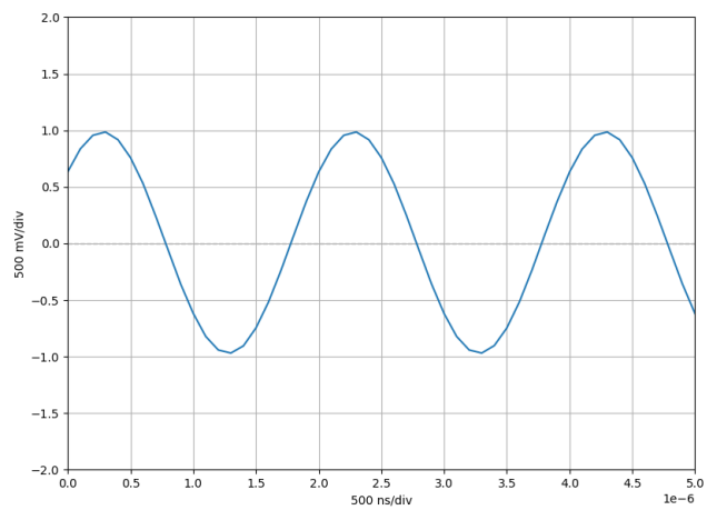
Abbildung 42: Testsignal: Sinus ( f = 500 \text{ kHz} , V_{pp} = 2 \text{ V} )
