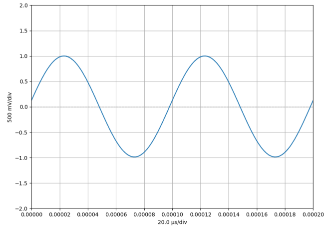
Abbildung 39: Testsignal: Sinus ( f = 10 \text{ kHz} , V_{pp} = 2 \text{ V} )
