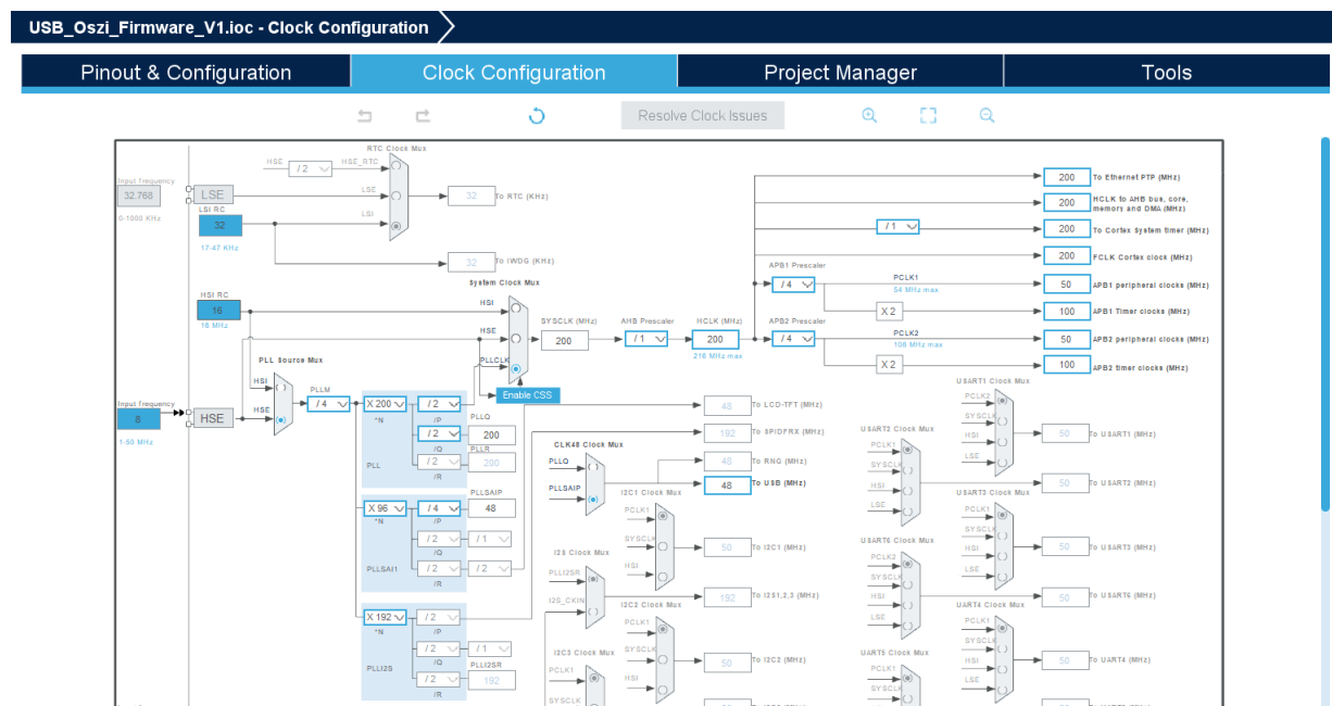
Abbildung 28: Clock-Tree-Ansicht in STM32CubeMX
