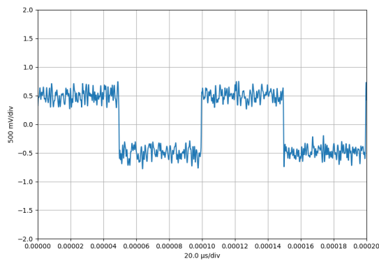
Abbildung 65: Signalverlauf ohne Filter 10kHz Rechtecksignal mit überlagertem Rauschen (1Vpp; Bandbreite: 1MHz)
