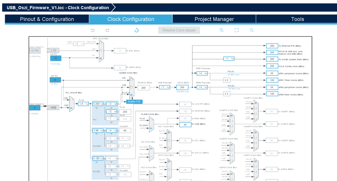
Abbildung 38: Clock-Tree-Ansicht in STM32CubeMX
