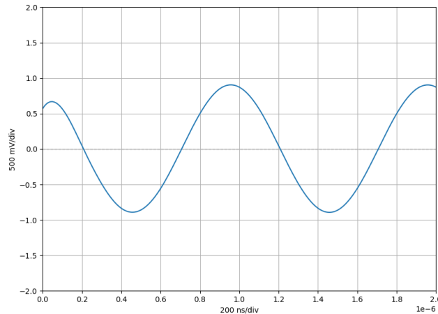
Abbildung 55: Testsignal: Sinus ( f = 1 MHz, V_{pp} = 2 V) Polynom-Interpolation
