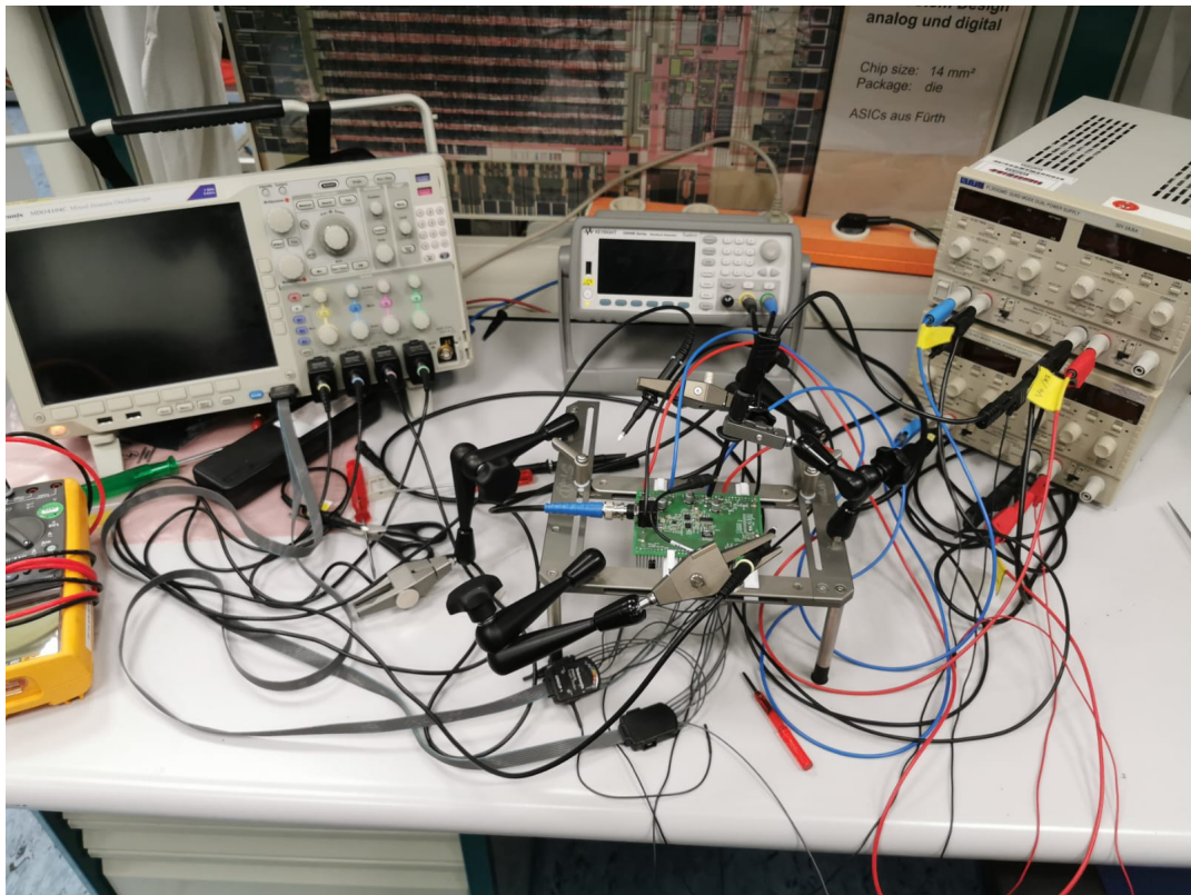
Abbildung 32: Aufbau zum Test der Hardware
