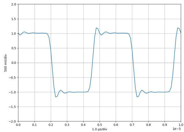
Abbildung 62: Testsignal: Rechteck ( f = 200 \text{ kHz} , V_{pp} = 2 \text{ V} )
