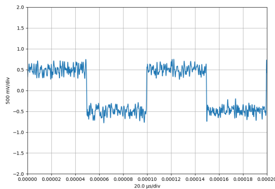
Abbildung 44: Signalverlauf ohne Filter 10kHz Rechtecksignal mit überlagertem Rauschen (1Vpp; Bandbreite: 1MHz)
