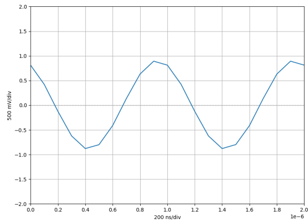
Abbildung 56: Testsignal: Sinus ( f = 1 \text{ MHz} , V_{pp} = 2 \text{ V} )
