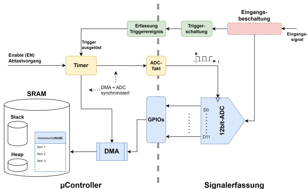
Abbildung 36: Funktionsschema der Abtastung
