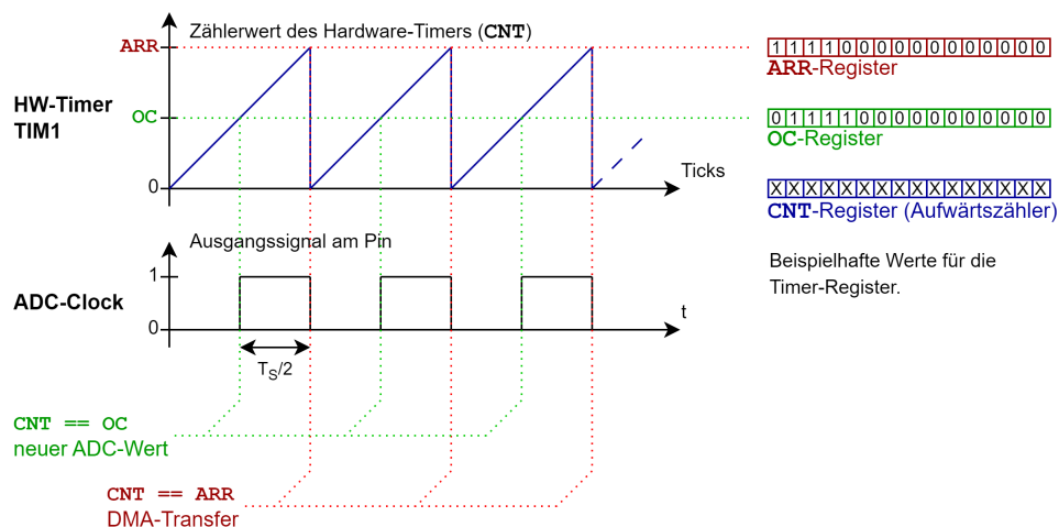
Abbildung 38: Zeitdiagramm und Registerübersicht des Hardware-Timers für die Synchronisation von ADC und DMA (Sampling am \mu\text{C} )
