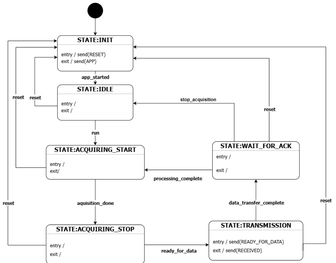
Abbildung 93: Statediagram PC
