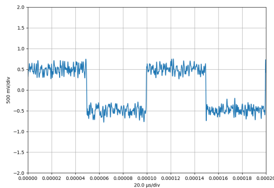
Abbildung 33: Signalverlauf ohne Filter 10kHz Rechtecksignal mit überlagertem Rauschen (1Vpp; Bandbreite: 1MHz)
