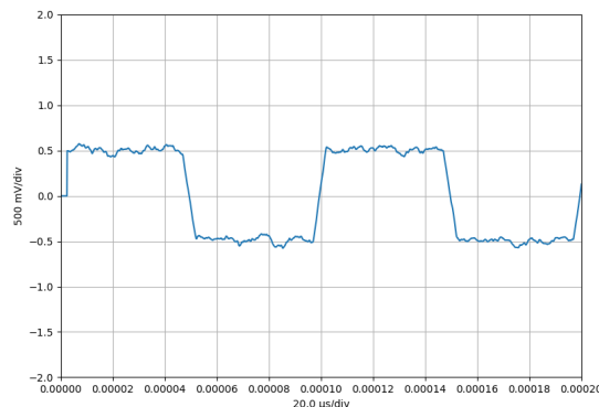
Abbildung 34: Signalverlauf rekursiver gleitender Mittelwertfilter (M=51) 10kHz Rechtecksignal mit überlagertem Rauschen (1Vpp; Bandbreite: 1MHz)
