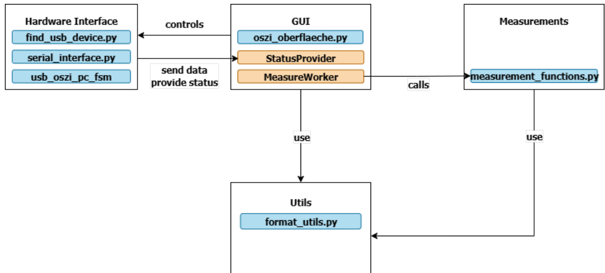
Abbildung 36: Paketdiagramm zur Darstellung der Unterprogramme
