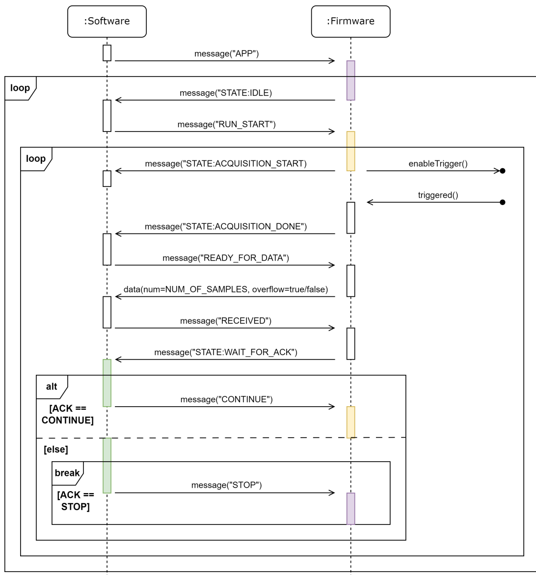
Abbildung 35: UML-Sequenzdiagramm: Kommunikation ohne Konfiguration
