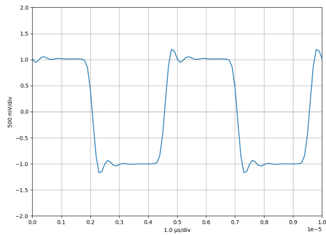
Abbildung 83: Testsignal: Rechteck ( f = 200 \text{ kHz} , V_{pp} = 2 \text{ V} )
