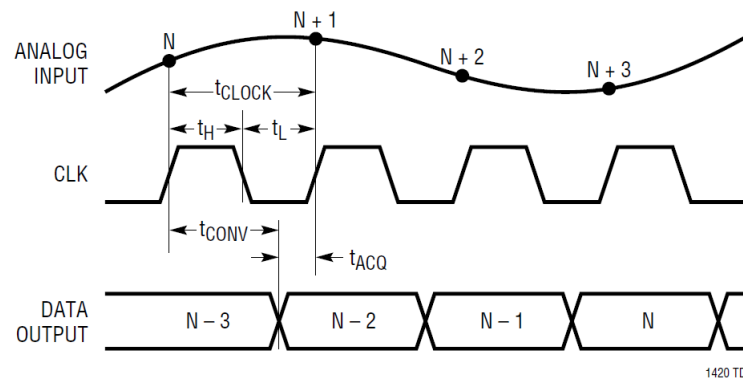
Abbildung 52: Timing Diagramm ADC aus [Linb, S. 7]
