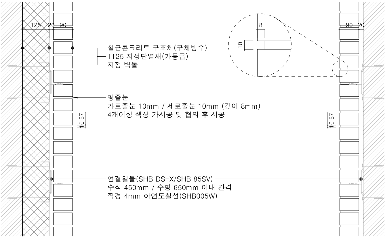
■ 길이 쌓기 시공 예시도
