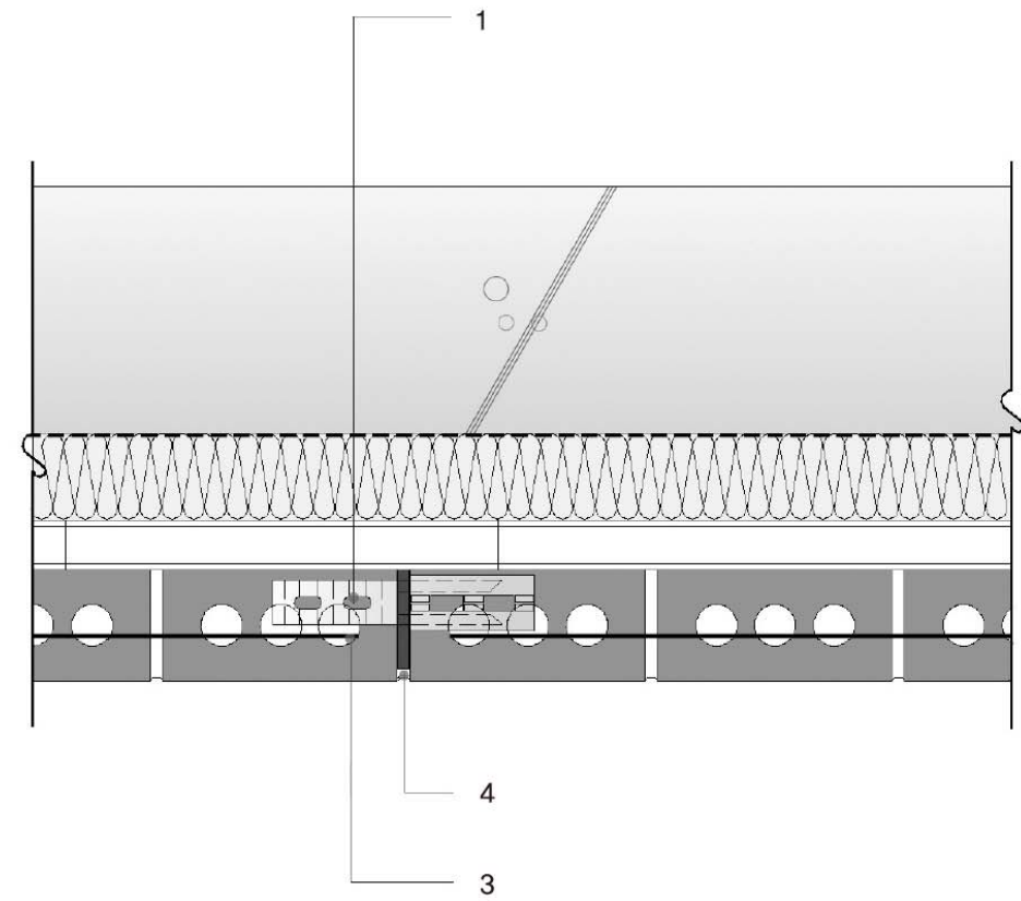
1.슬립세트 SHB JS-1 2.수직팽창조인트 SHB JOINT 3.아연도철선 SHB 005W 4.코킹마감
