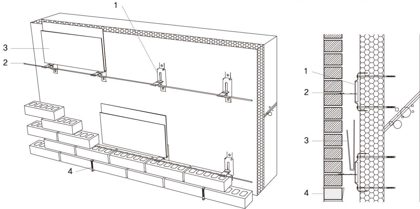
SHB DS-X 수직450mm 수평650mm간격
