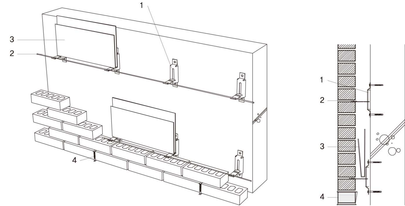
SHB DS-C 수직450mm 수평650mm간격
