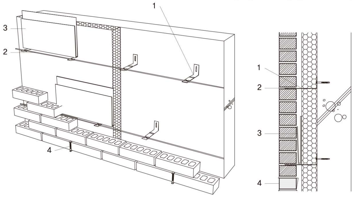
SHB 170L 수직400mm 수평900mm간격
