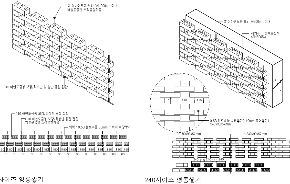
■ 영롱쌓기_옥탑층 난간
