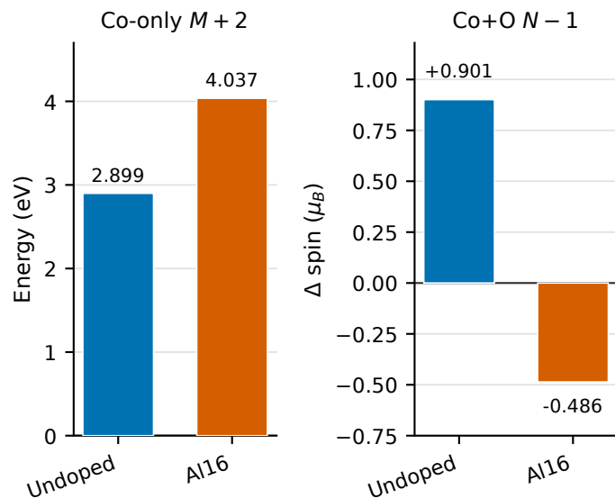
(d) Constrained-state fingerprints for *O
