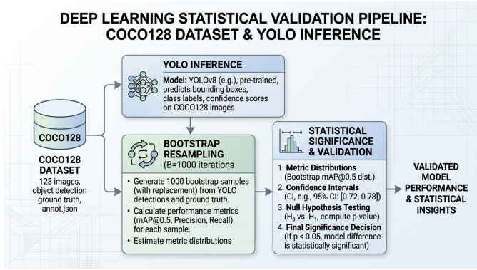
Figura 1. Pipeline automatizado de validación estadística para YOLO.
