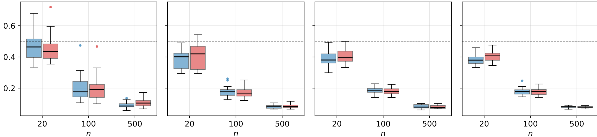
relative Procrustes error
