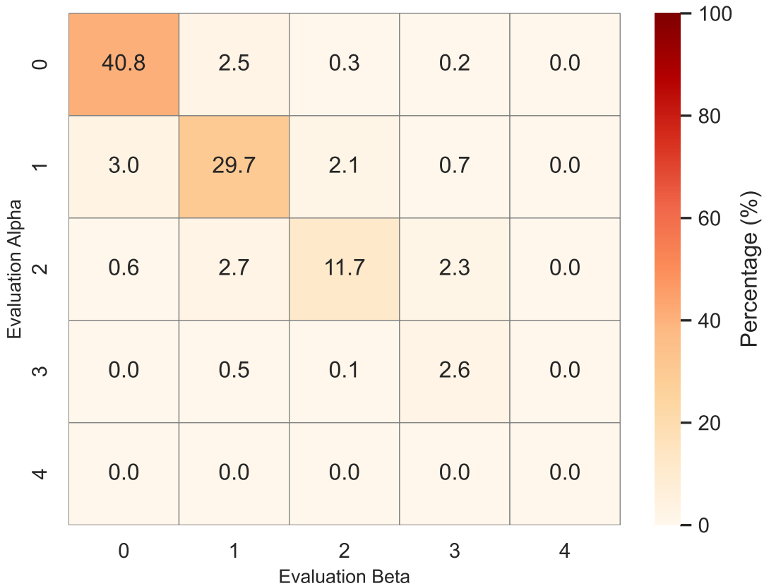
Gemini3pro
