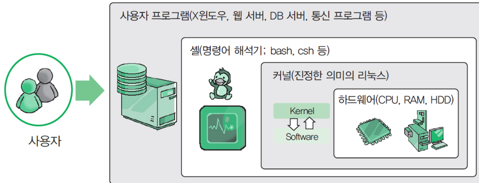
그림 1-2 리눅스의 커널과 셸, 사용자 프로그램의 관계
