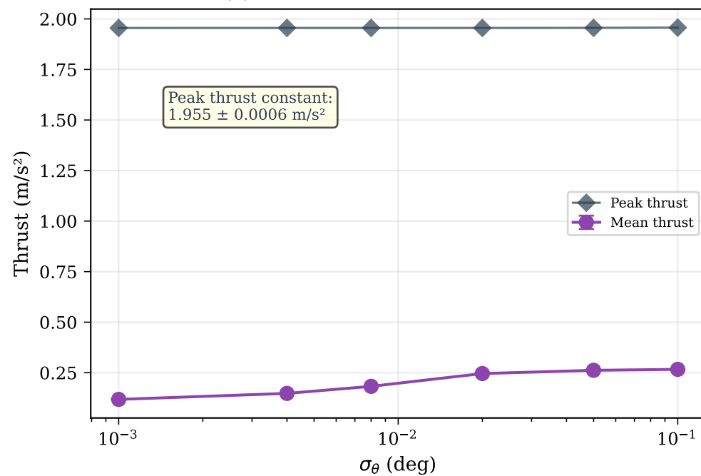
(d) Thrust statistics vs. sensor noise
