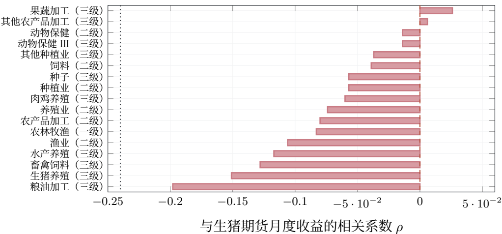
图 6-8 申万农业子行业指数与生猪期货的月度收益率相关系数（1 个一级、6 个二级与 10 个数据可得的三级行业指数；主窗口 67 个月度点，全部未达 5% 显著性阈值 |\rho| > 0.24 ）
