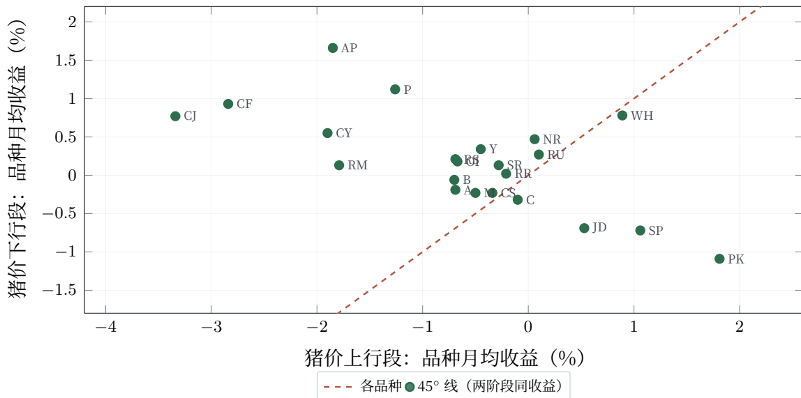
图 6-6 生猪价格上行段与下行段中，各期货品种的月均收益率（上行段 15 个月、下行段 47 个月；点位于 45° 线上方说明该品种在猪价下跌时表现更好）
