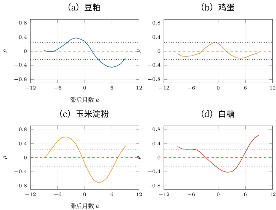
图 6-4 与生猪周期分量的领先滞后互相关（ k > 0 表示该品种滞后猪周期 k 个月；点线为 5% 双侧显著性阈值 \pm 0.24 ，仅绝对值超过该阈值的滞后阶视为显著）
