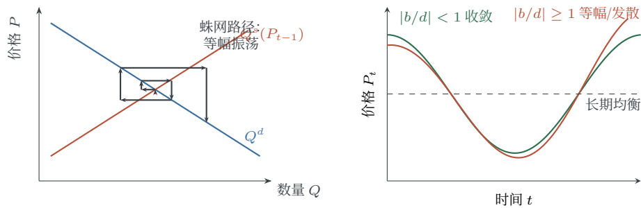
图2 蛛网模型：供给时滞下的价格振荡（左）与振荡幅度演化（右；参数 b/d 取 0.7 与 1.045）
