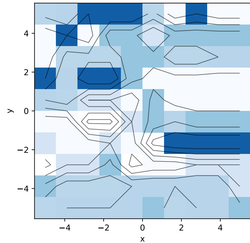
(a) EDC clusters — est. b
