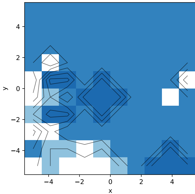
(b) LEC clusters — est. b
