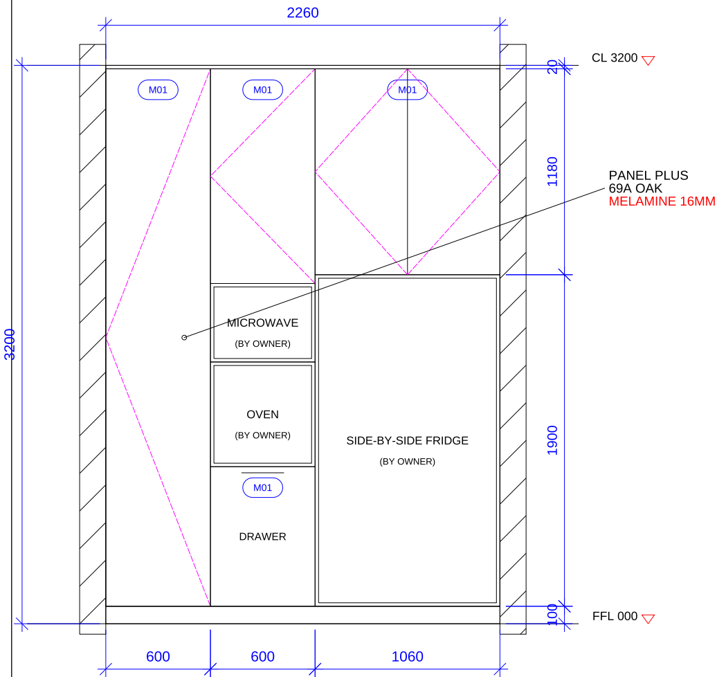
ELEVATION A 1:30
