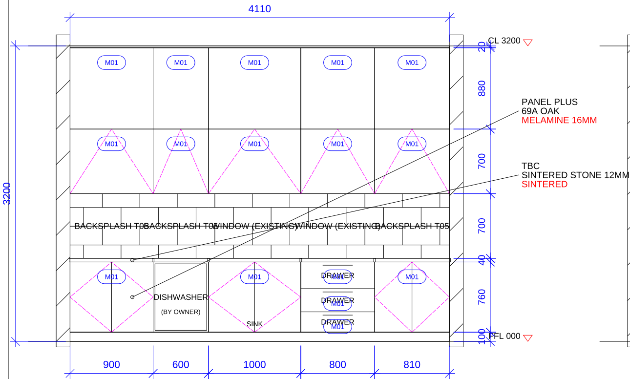
ELEVATION A 1:40
