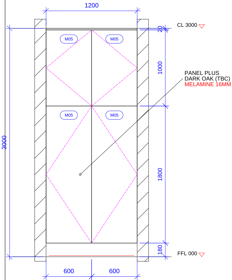
ELEVATION A 1:30
