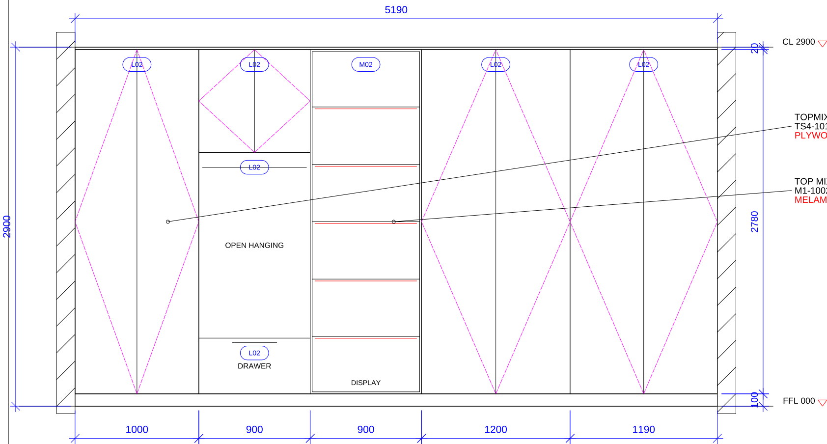
ELEVATION A 1:30
