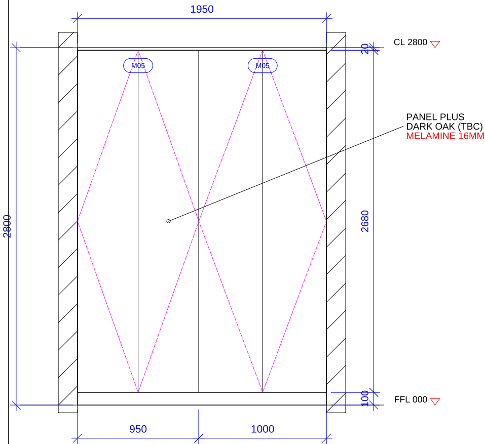
ELEVATION A 1:30
