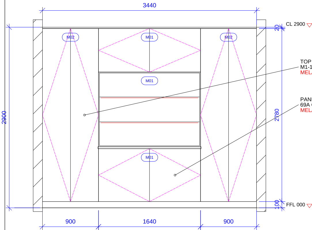
ELEVATION A 1:35
