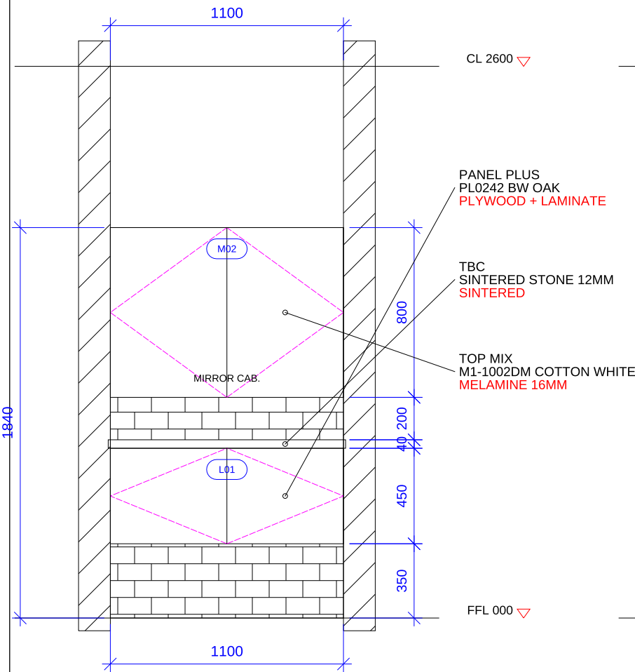
ELEVATION A 1:25
