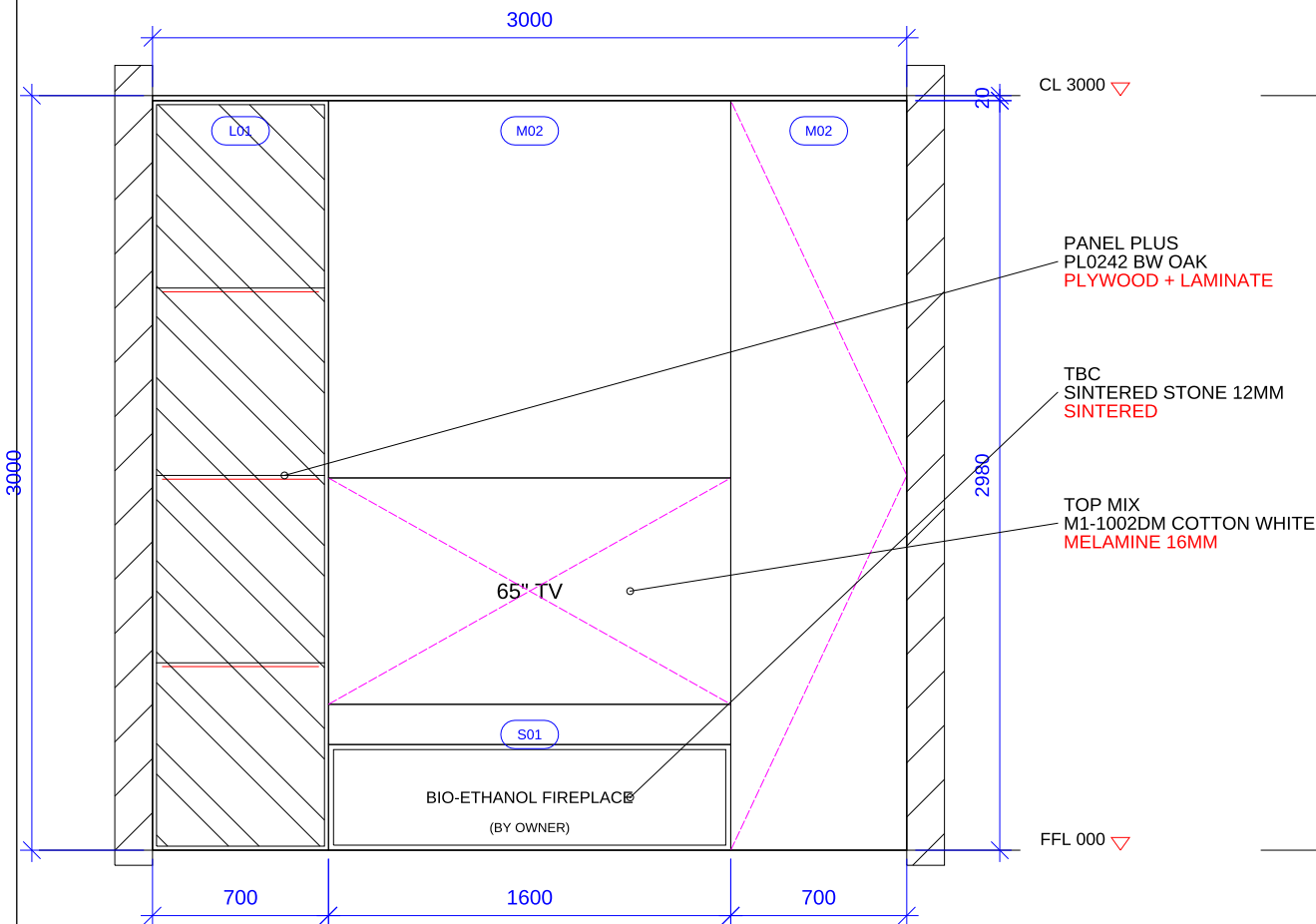
ELEVATION A 1:30
