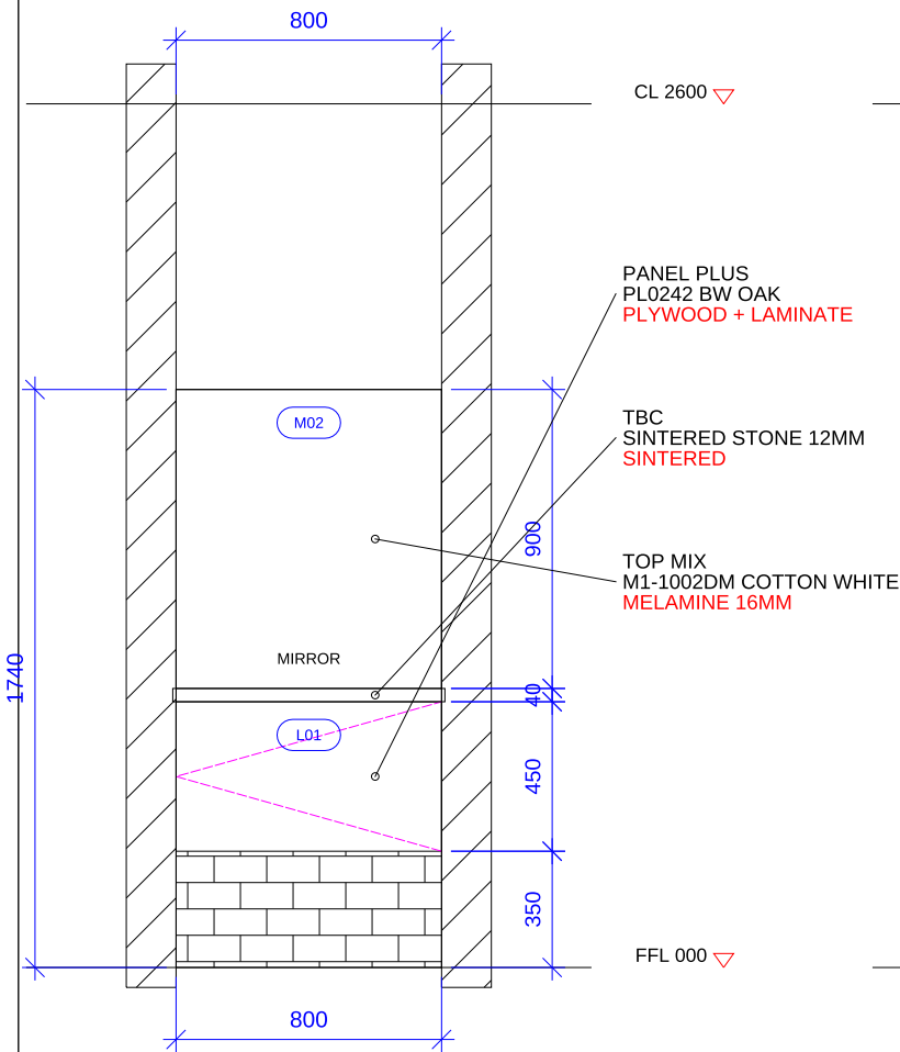
ELEVATION A 1:25
