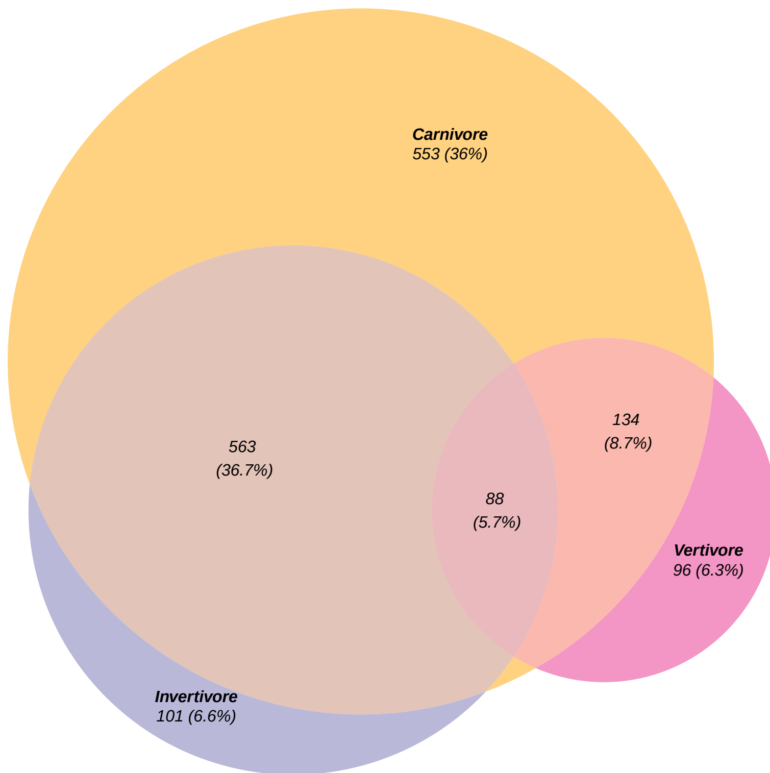
Genes (p.adj < 0.05)
