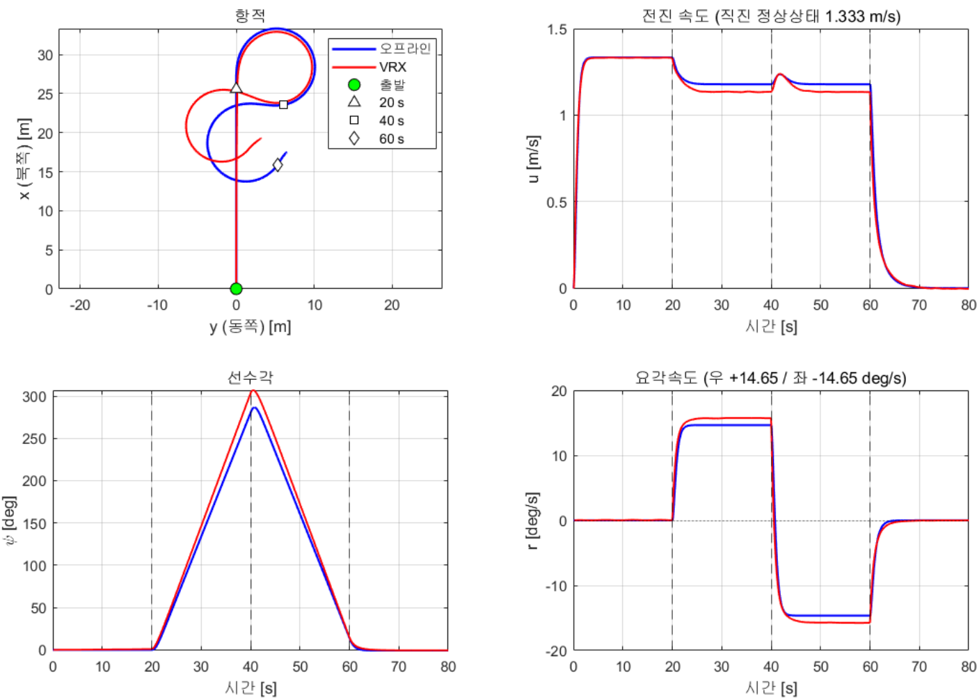
W04 5단계 — 오프라인 WAM-V(파랑) vs VRX(빨강)
