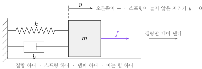
① 장치
