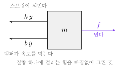
② 자유물체도
