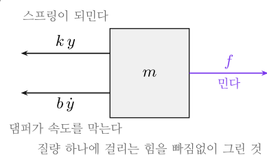
② 자유물체도
