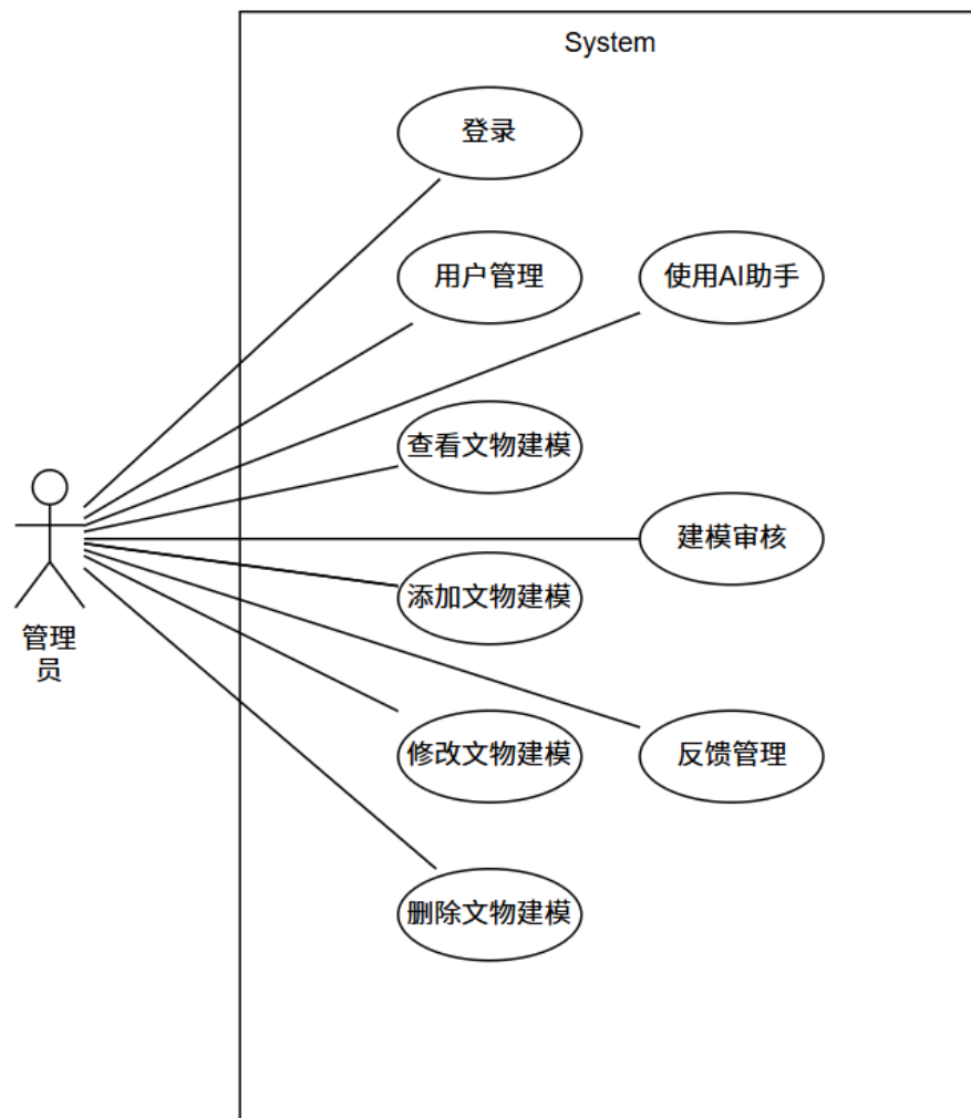
图2-5 管理员用例图
