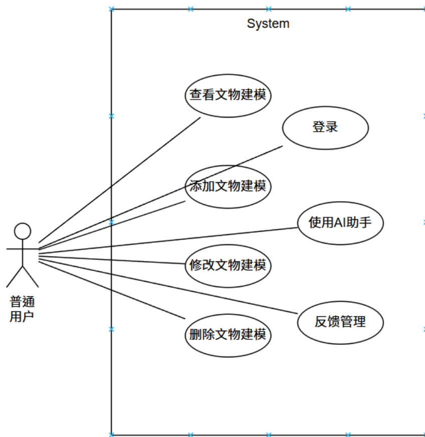
图2-3 普通用户用例图
