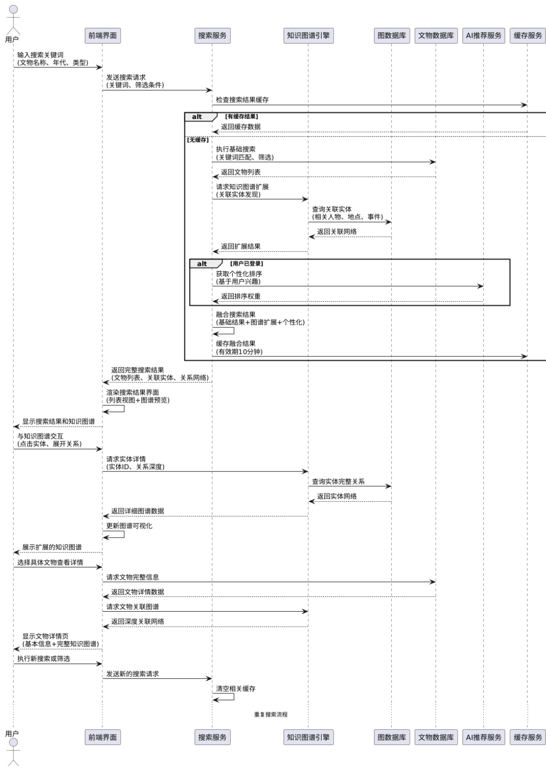
智能搜索与知识图谱展示时序图
