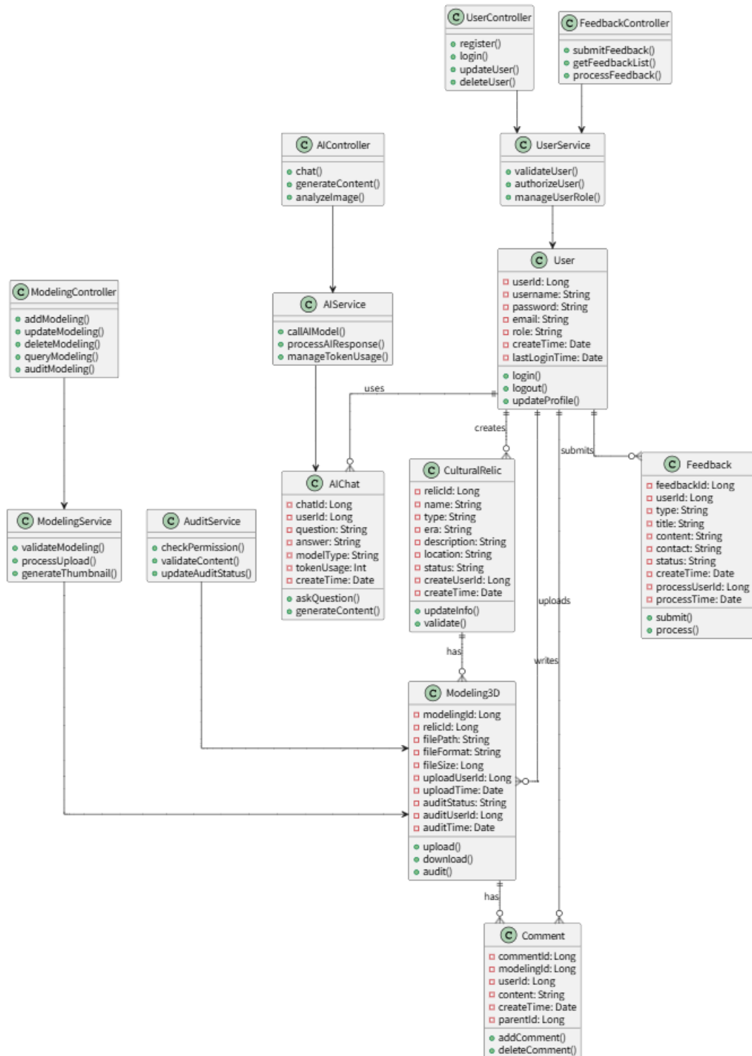
图3-1 大模型增强的文物资源知识管理系统类图
