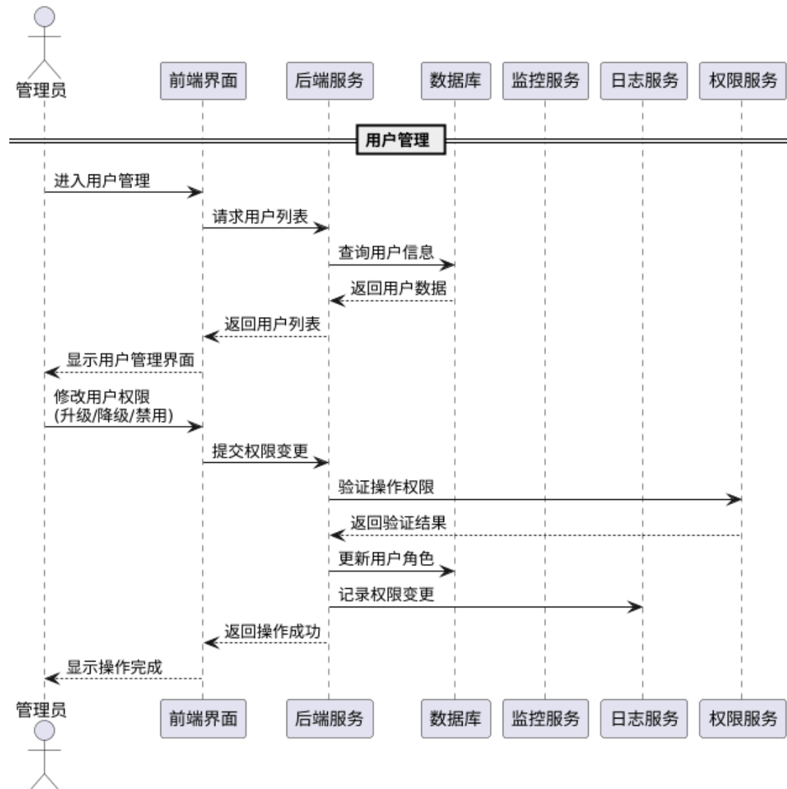
系统管理时序图
