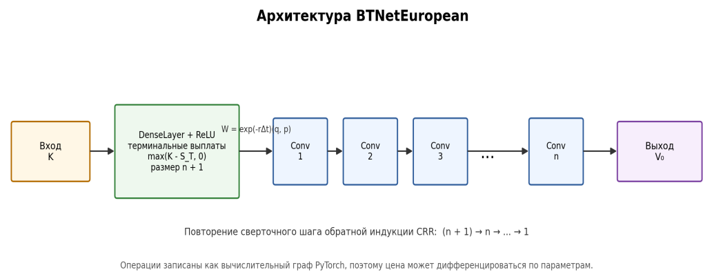
Рисунок 2.1 – Архитектура модели BTNetEuropean
