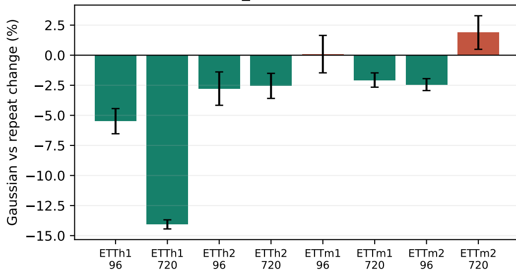
no_attention / MSE
