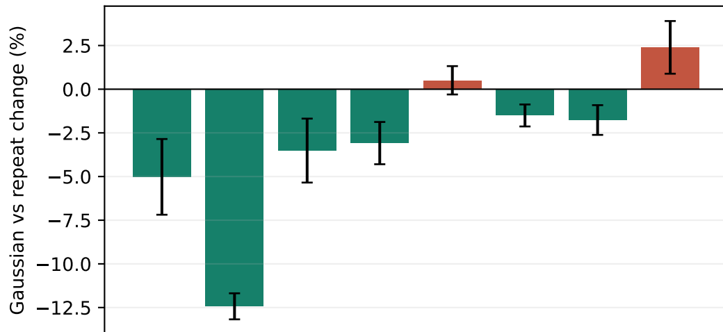
temporal / MSE
