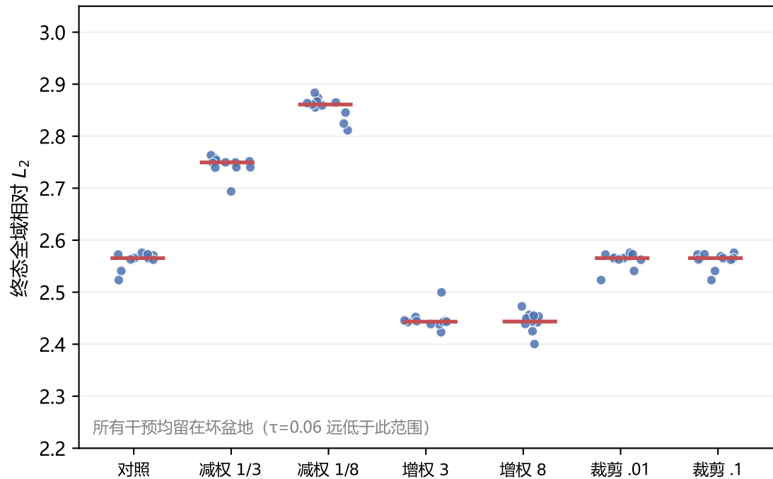
(b) caseB 人为坏盆地: 减权与裁剪均救不出
