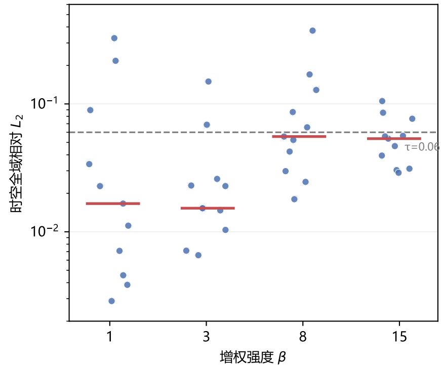
(a) D1 时变 Burgers (有理族) : 各档无显著差异
