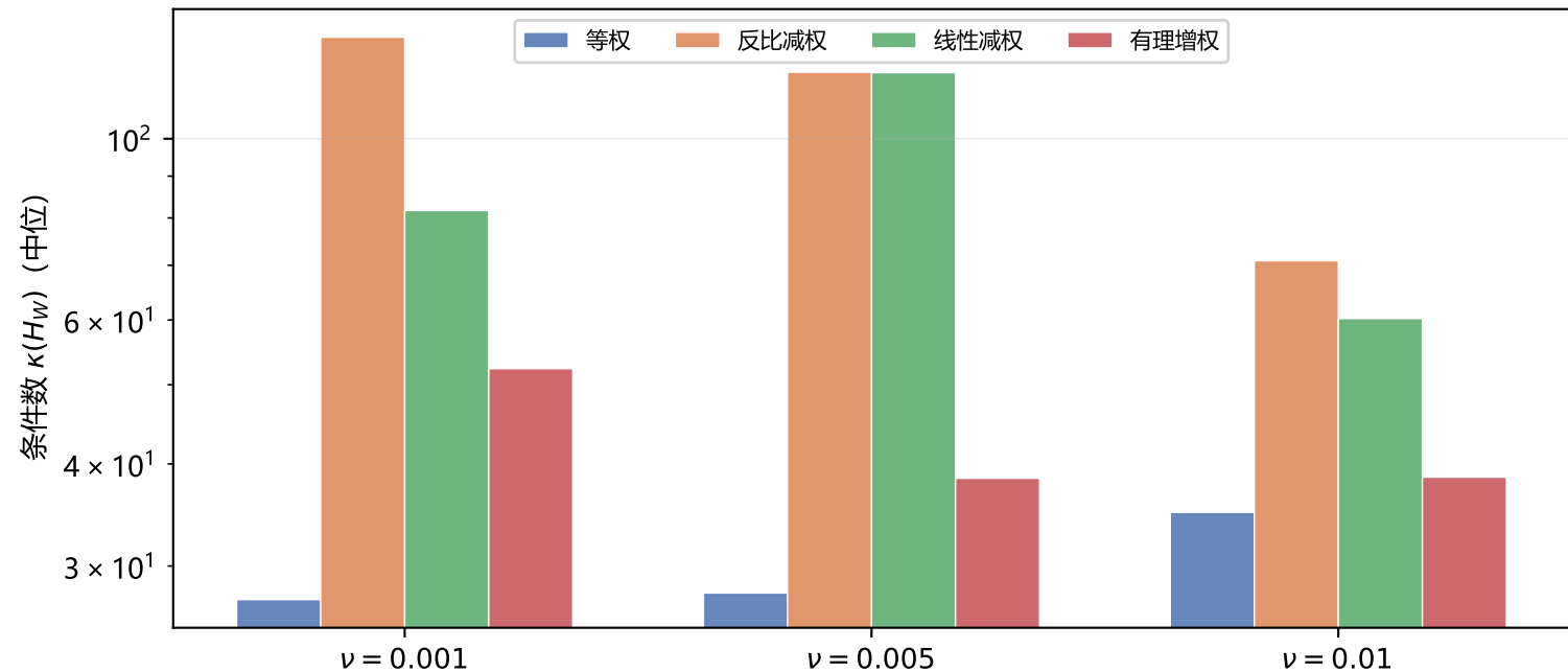
Gstab: 各权重族条件数 (静态 Hessian 近似)
