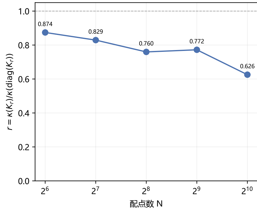
F1d: 真实 Burgers Jacobian 上局部对角权的谱能力
