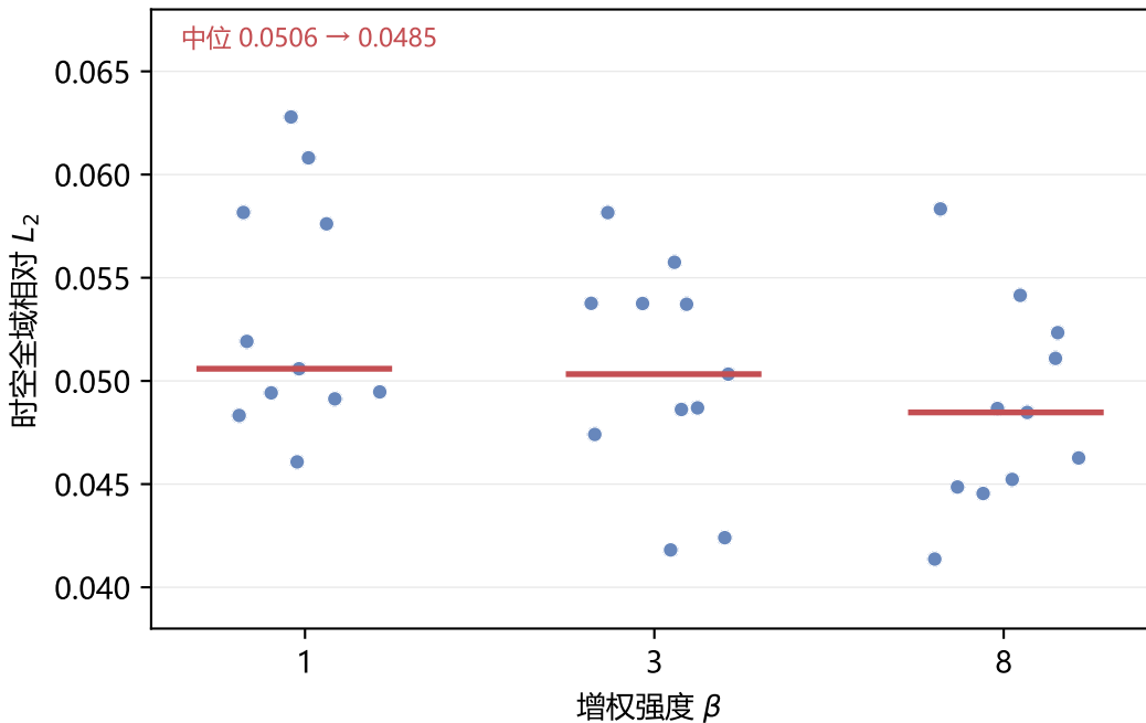
C4/C5 二维线性对流—扩散：33 个 run 全部进入好盆地
