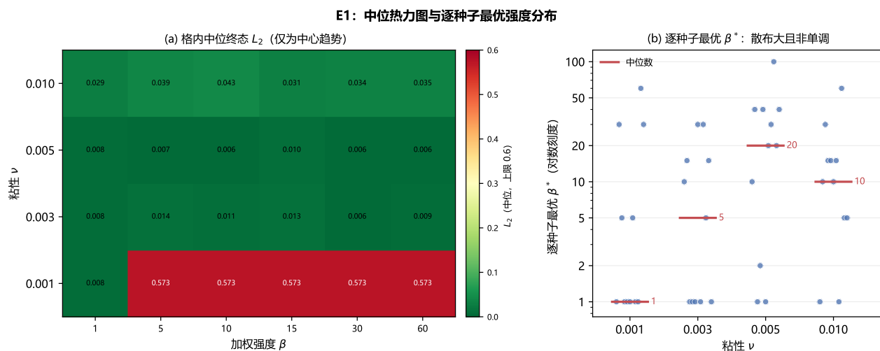
图 7: 实验 5.4: 左: 格内中位终态 L_2 ( n = 11 , 仅显示跨种子中心趋势) 随加权强度 \beta 与粘性 \nu 的变化; 右: 逐种子最优 \beta^* 分布 (各 \nu 中位 1/5/20/10、整体中位 10, 范围 [1, 100] )。薄激波端存在事后最优 \beta , 但逐种子散布大且不随粘度单调; 格内中位数最小点与逐种子 \beta^* 中位数不必一致, 本图不用于识别可部署策略。大粘性端曲线近平坦、相对增益落误差地板。左图仅显示四个粘度公共的 6 档 \beta ( \nu = .005 的加密档见附录表 8); \nu = .001 、 \beta \geq 5 各深红格为全部种子塌缩到的同一失败态 (格内中位 \approx .573 )。
