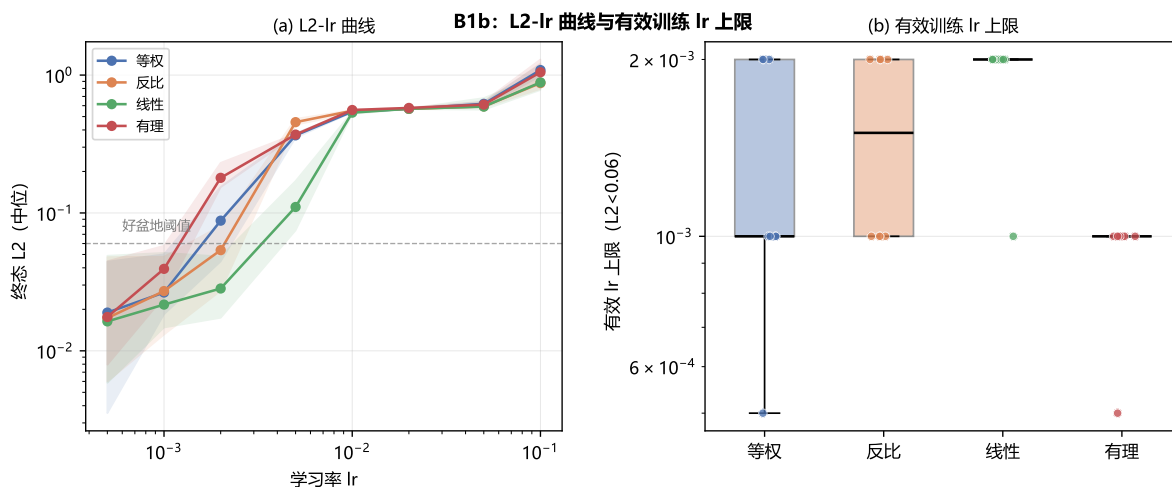
图 8: 实验 5.8: 盆地内 lr 裕度 ( n = 8 配对, 从 Gate 点出发固定步长 Adam 500 步)。左: 终态 L_2 随 lr 的变化 (中位 \pm IQR ), lr \geq .01 四族全部平台化 (离开好盆地), 虚线为好盆地阈值 L_2 = .06 ; 右: 以 L_2 < .06 定义的有效训练 lr 上限箱线图, 线性减权 down_lin 中位 .002 高于等权 uniform .001 (配对 Wilcoxon 精确双侧 p = .0625 、渐近 \approx .043 , 方向一致但未达 .05 显著的边缘趋势)。
