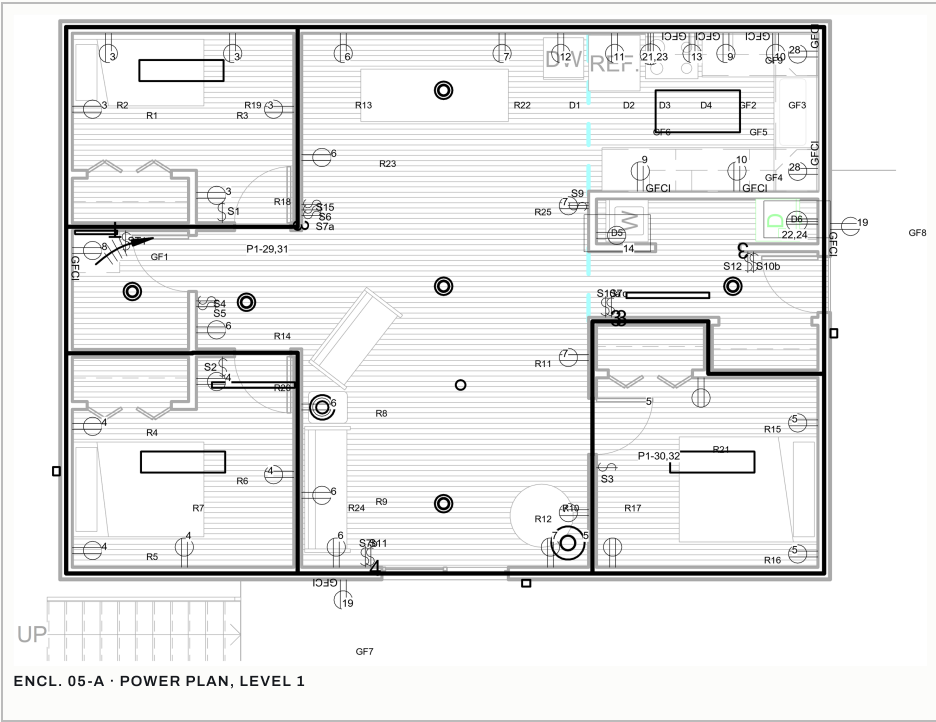
ENCL. 05-A · Power plan, Level 1
