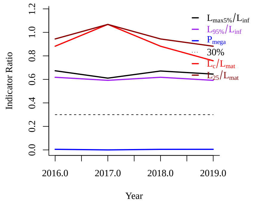
(d) Optimal yield
