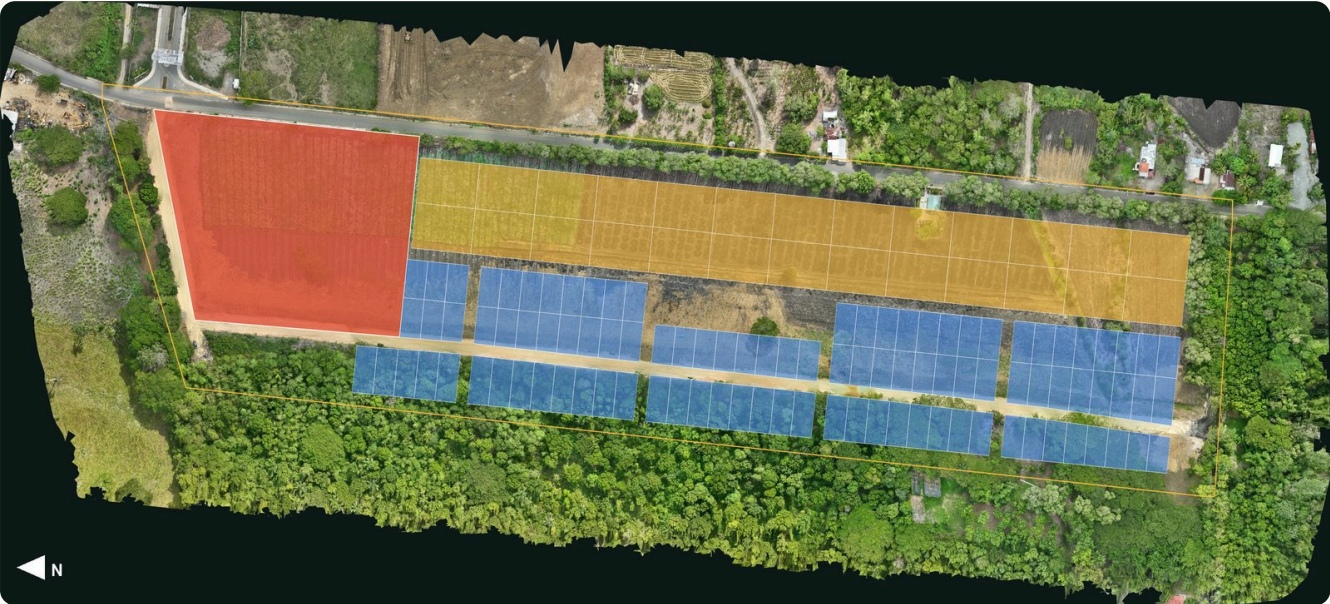
La distribución del DXF sobre la ortofoto del vuelo de dron (4 cm por píxel), con el norte a la izquierda. Rojo: solar comercial. Amarillo: mixtos. Azul: residenciales. Línea naranja: envolvente del dibujo.
