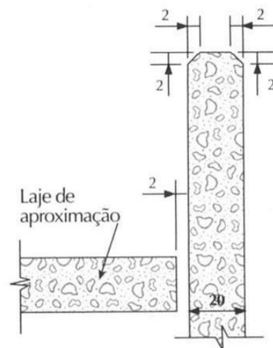
Detalhe da junta de pavimentação
