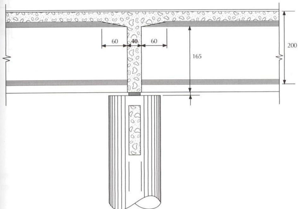
Transversina de apoio — detalhe
