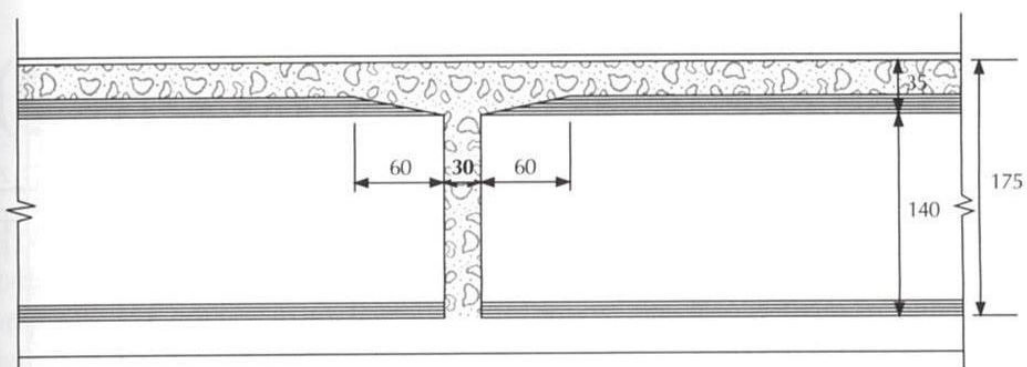
Transversina de vão — detalhe
