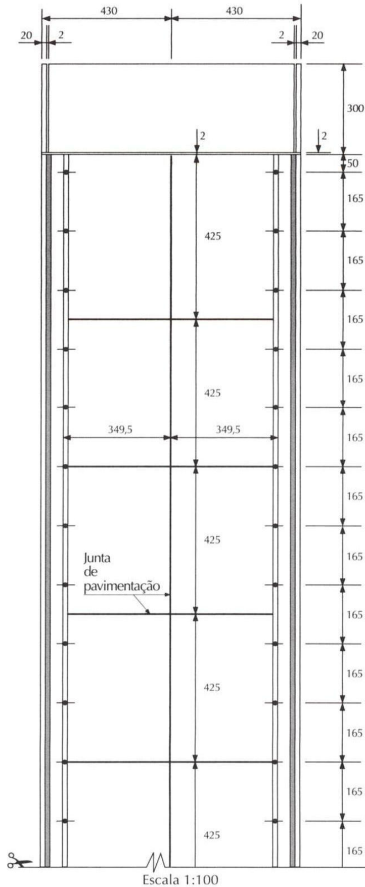
1/2 Planta do tabuleiro
