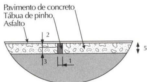
Detalhe da junta de pavimentação
