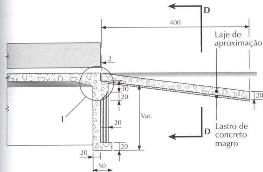
Detalhe das abas
