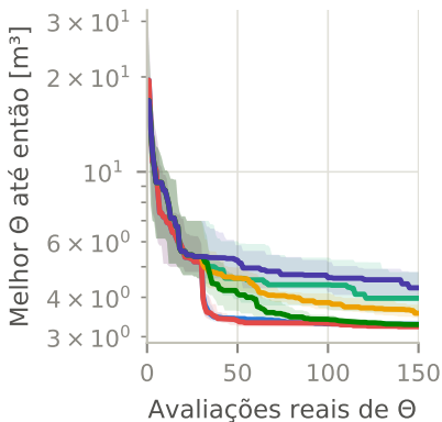
Caso 1 — 1 sapata (dim. 3)
