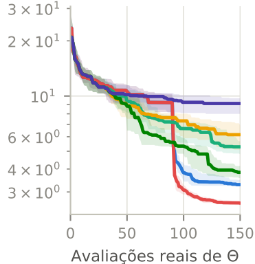
Caso 3 — 3 sapatas (dim. 9)
