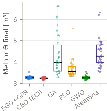
Caso 1 — 1 sapata (dim. 3)
