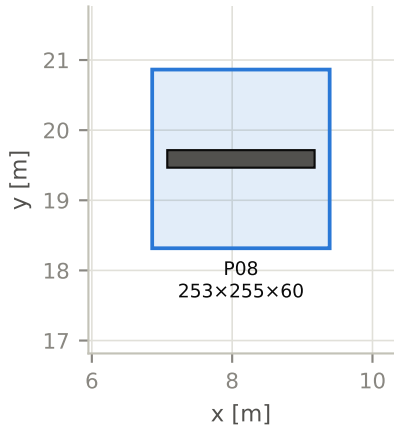
Caso 1 — 1 sapata (dim. 3)
