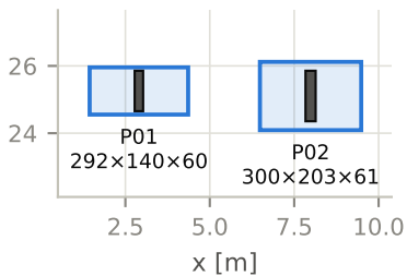
Caso 2 — 2 sapatas (dim. 6)
