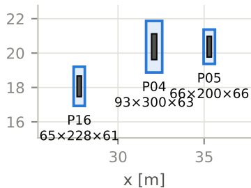
Caso 3 — 3 sapatas (dim. 9)
