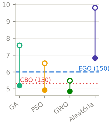
Caso 2 — 2 sapatas (dim. 6)
