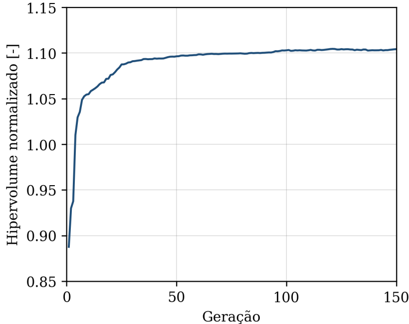
Figura 9: Evolução do hipervolume ao longo das gerações do NSGA-II.
