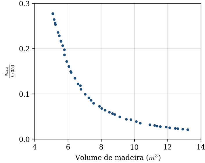
Figura 8: Fronteira eficiente da célula de referência C-13 ( L = 5,0 m, D40, \rho = 5\% ).
