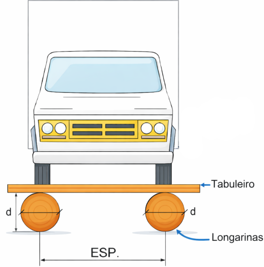
Figura 3: Representação conceitual do sistema estrutural da ponte de madeira.
